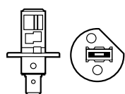
P14,5s IEC 7004-46
